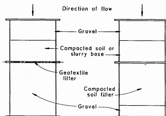
(a) Acrylic Cylinder System (subpar. 8.2.1.1)
