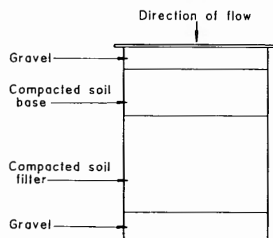
(b) Aluminum Cylinder System (subpar. 8.2.1.2)
